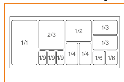
Gastronorm maatvoering
